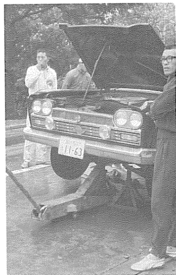
セドリックG30のクラッチペダルの修理。
